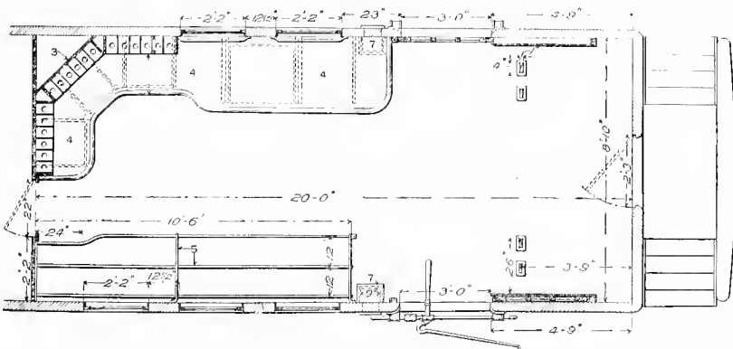
Fig. 615. Sectional Plan.
